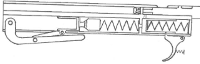
3. ábra – Pneumatikus rendszerű
