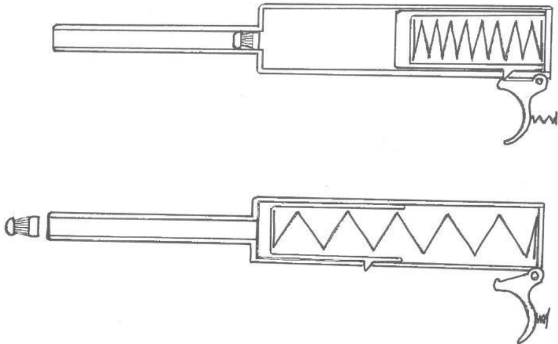
7. ábra –Lövedék előre mozgása a fegyvercsőben
