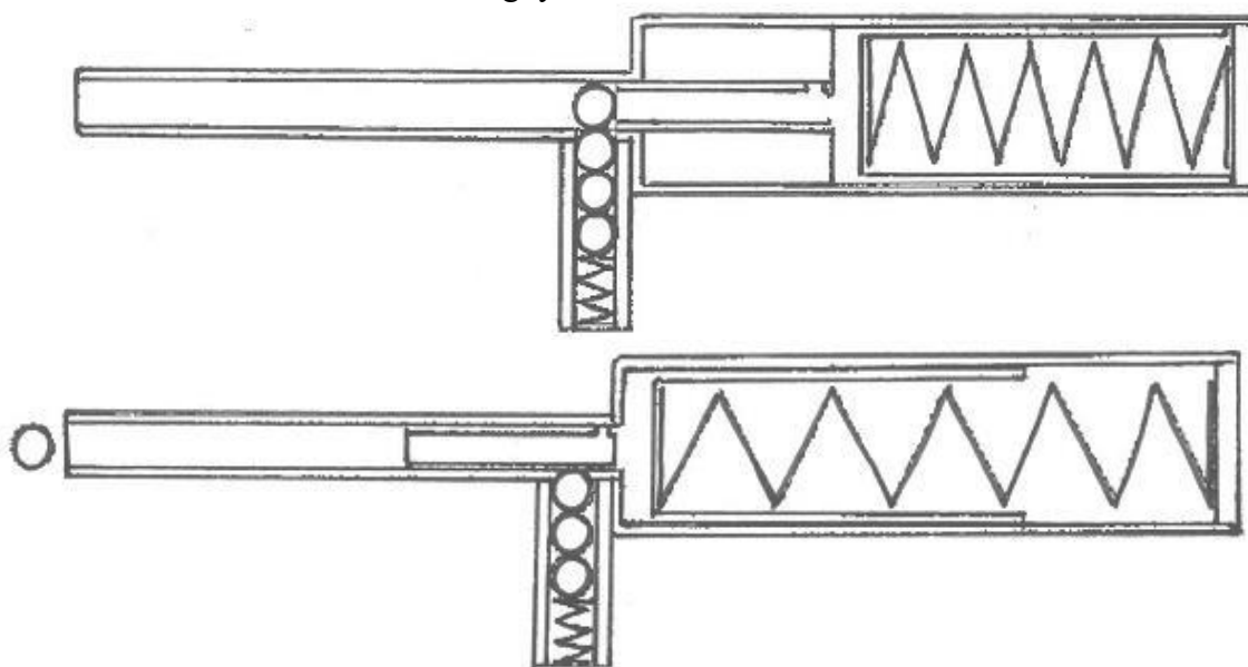
10. ábra – Lövedék kilövésének folyamata
