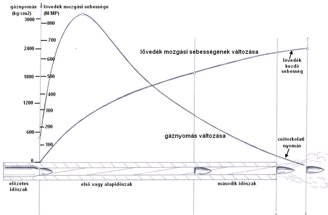
11. ábra – A lövés folyamata
