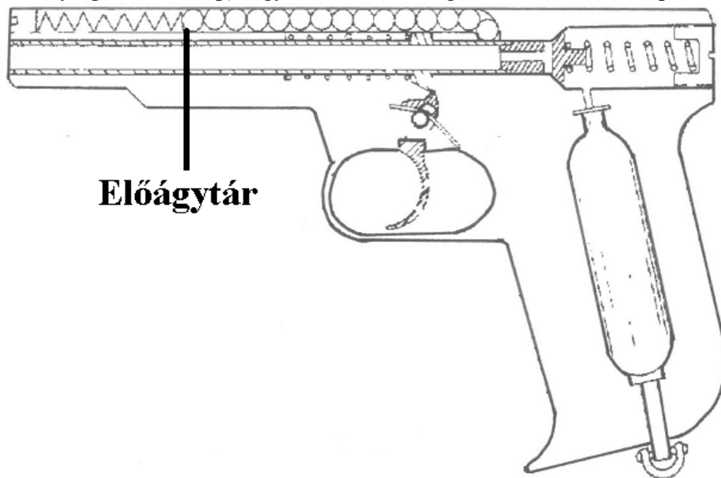
9. ábra – Ismétlő rendszerű légfegyver
