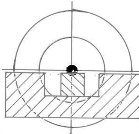
17. ábra – Célzás nyílt irányzékkal
