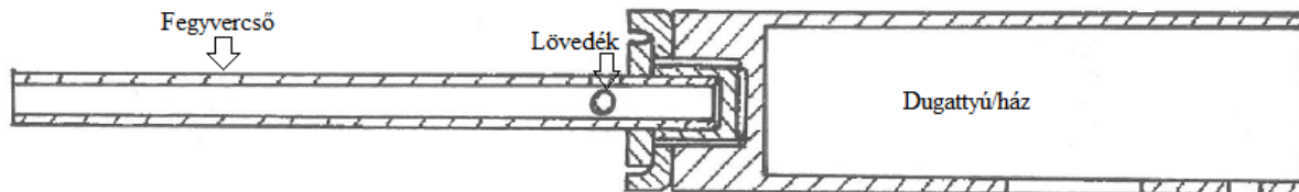
8. ábra – Dugattyúház és fegyvercső
